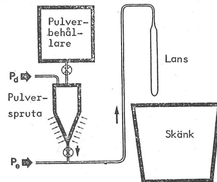
Principskiss av anordning för pulverinjektion med lans
