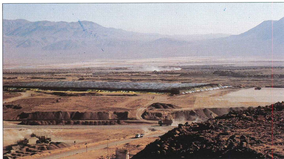
Kopparmalmen lakas ut inom stora invallningar
